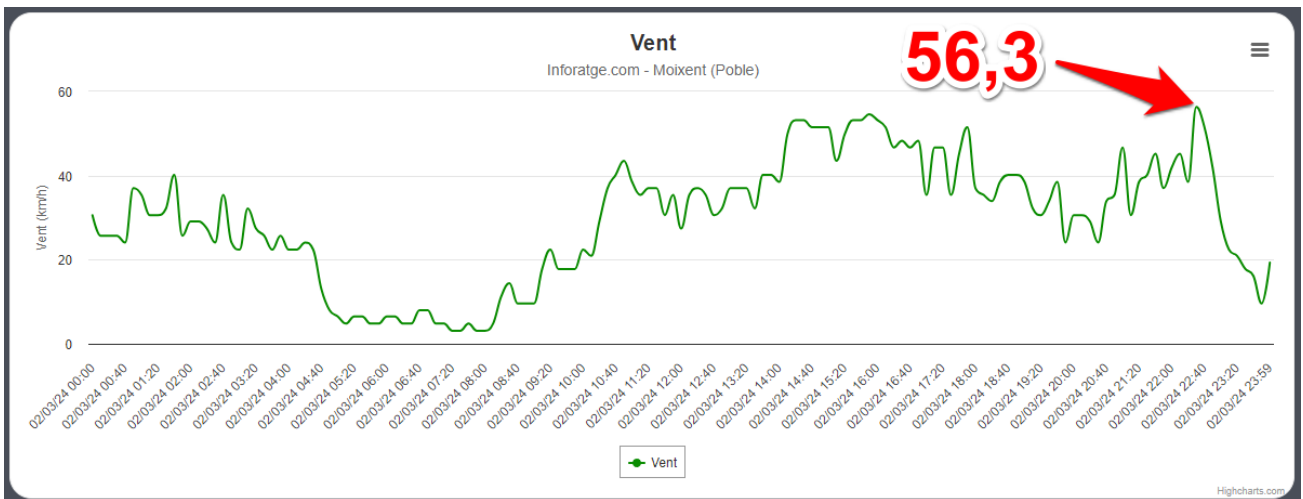
Ráfagas de viento registradas en MOIXENT (núcleo urbano) el 02/03/24 (en km/h) https://inforatge.com/meteo-moixent
