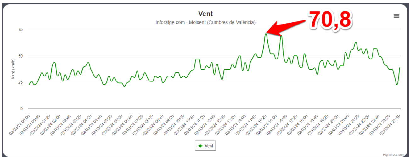
Ráfagas de viento registradas en MOIXENT (Cumbres de València) el 02/03/24 (en km/h) https://inforatge.com/meteo-moixent
